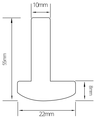
T-LIPPING DOOR DIVIDER 55 x 22
